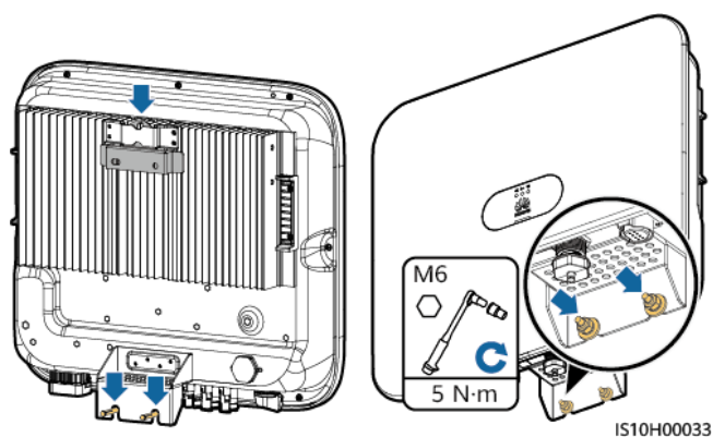
Figure 4-11 Installation av SUN2000
