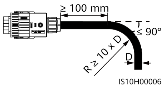
Figure 5-10 Kabelriktning
