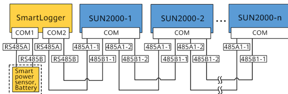
Figure 5-20 Nätverk med SmartLogger (den streckade rutan anger valfria komponenter)
