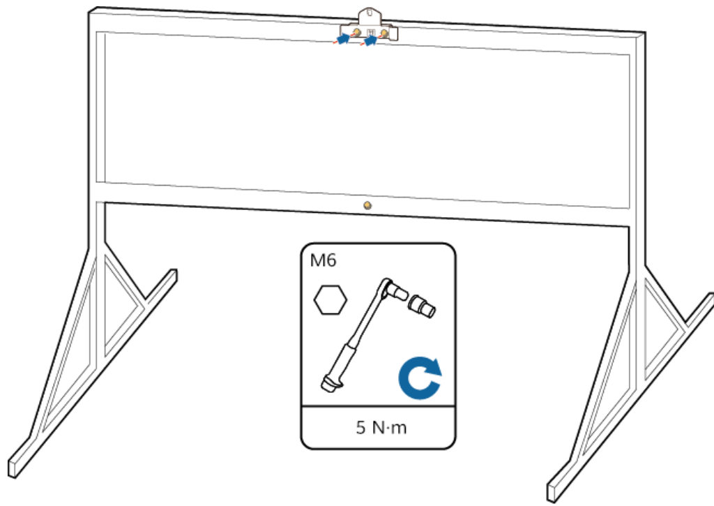
Figure 4-15 Att säkra monteringsfästet
