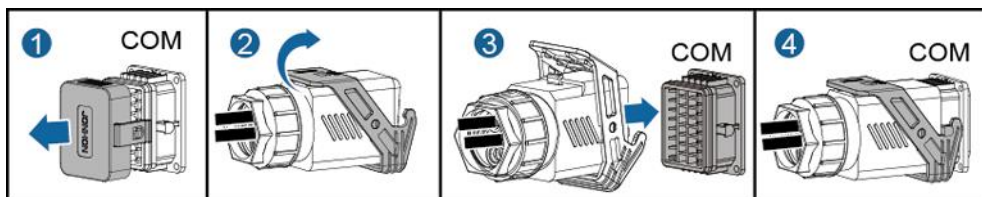
Figure 5-28 Säkra signalkabelns kontakt
